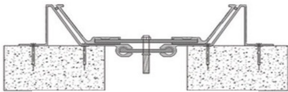
Seismic Pan Type EJ
