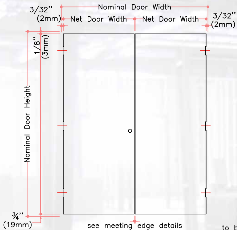
Double Door Elevation
