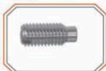
SLOTTED SET SCREWS DOG POINT DIN 417
