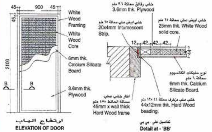
الشكل ٢ : باب مقاوم للنار ساعة واحدة TYPE - 2 : ONE HOUR FIRE RATED FLUSH DOOR
