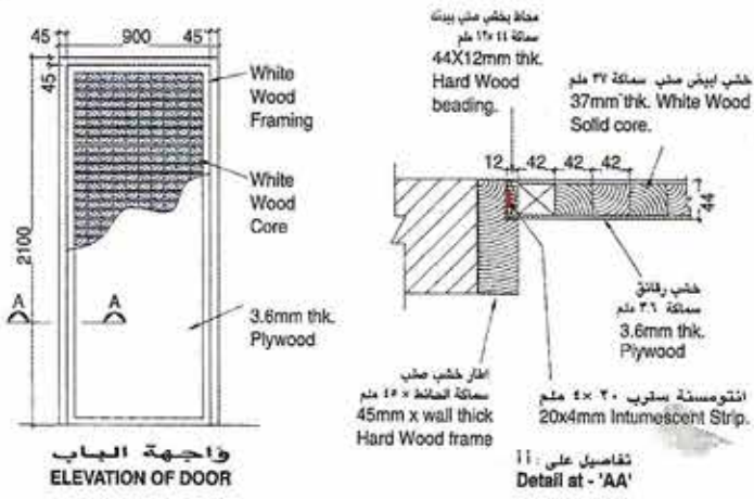
الشكل ١ : باب مقاوم للنار نصف ساعة TYPE - 1 : HALF HOUR FIRE RATED FLUSH DOOR
